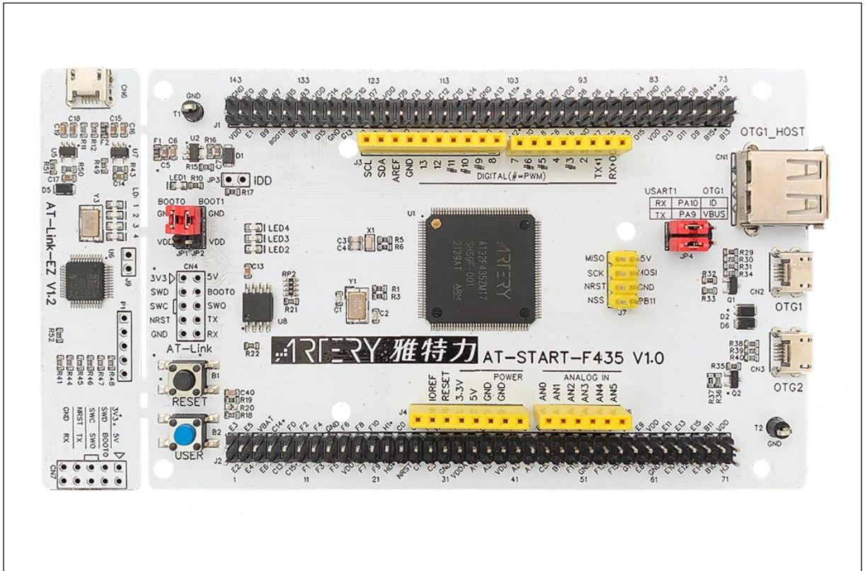
图 1. AT-START-F435 V1.0 开发板
